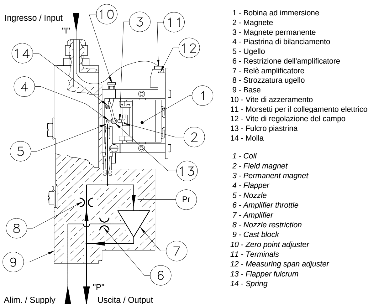
Fig. 1 - Schema funzionale / Schematic diagram
